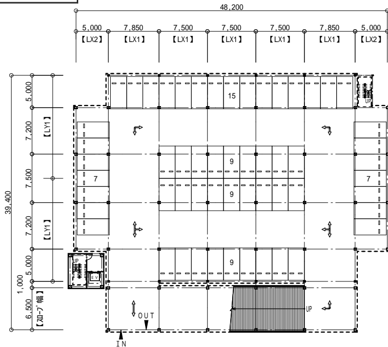
1階 平面図
