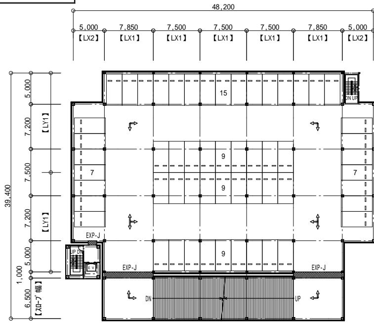
2～3階 平面図
